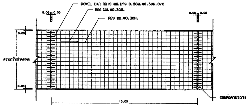
แบบแสดงการเสริมเหล็กถนนคอนกรีตเสริมเหล็ก NOT TO SCALE
